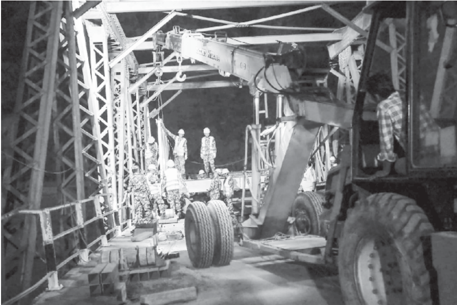
बेलिब्रिज जडानमा सेना: सिन्धुलीको खुर्कोट र रामेछापको मन्थली जोड्ने पक्की पुलको आधा भाग सुनकोशी नदीमा आएको बाढीले बगाएपश्चात् पुनर्निर्माणमा खटिएका नेपाली सेनाको टोलीद्वारा जडान गरिएको बेलिब्रिज । यो कार्य सम्पन्नसँगै मंगलबारबाट यातायात सुचारु भएको छ ।
